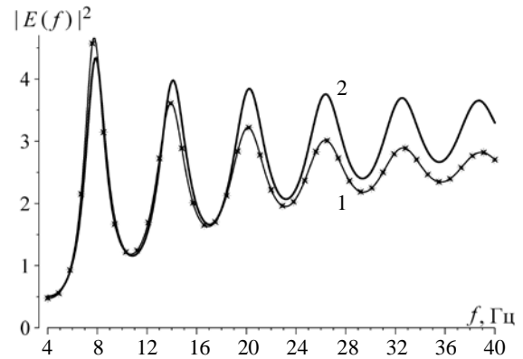
Рис. 3. Энергетические спектры вертикального электрического поля, рассчитанные при однородном распределении мировых гроз по Земле. Кривая 1 – точное решение для профиля 1; кривая 2 – решение, полученное для того же профиля, но в рамках эвристического подхода [31]
