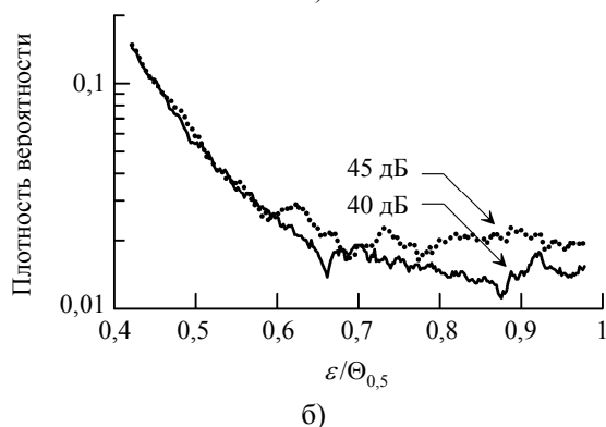
Рис. 4. Распределения измеренных углов места при различных отношениях сигнал/шум ( M = 5 ; \rho_d = 0,10 ; p = 5 ): а) распределения вблизи направления на цель; б) «хвосты» распределений для S/N = 40 и 45 дБ
