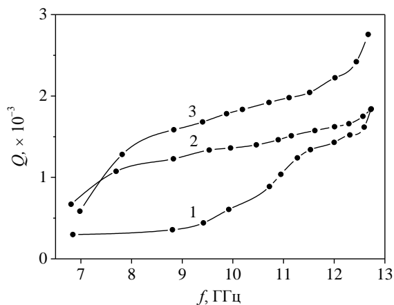
Рис. 6. Графики зависимости добротности ВКР № 2 и № 3 от частоты при перестройке КЗ-поршнями разных типов: кривая 1 – перестройка ВКР № 2 простым КЗ-поршнем; кривая 2 – перестройка ВКР № 2 РКЗ-поршнем; кривая 3 – перестройка ВКР № 3 РКЗ-поршнем
