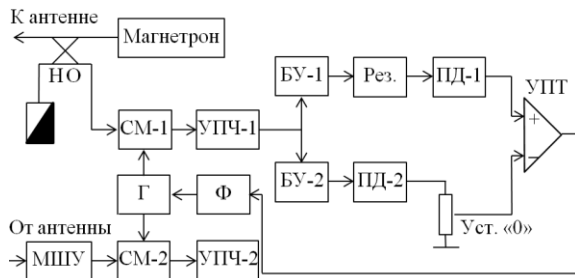
Рис. 1. Функциональная схема системы автоматической подстройки частоты: НО – направленный ответвитель; СМ-1, СМ-2 – смесители; МШУ – малошумящий усилитель; УПЧ-1, УПЧ-2 – усилители промежуточной частоты; Г – гетеродин; Ф – фильтр; БУ-1, БУ-2 – буферные усилители; Рез. – полосковый резонатор; ПД-1, ПД-2 – пиковые детекторы; УПТ – операционный усилитель; Уст. «0» – резистор
