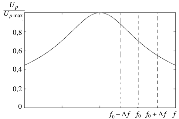
Рис. 2. Амплитудно-частотная характеристика резонатора
