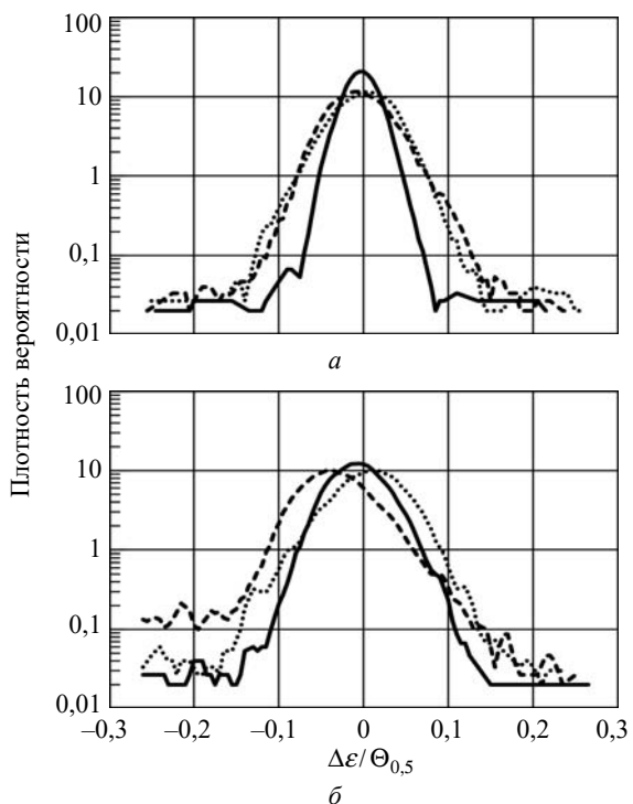
Рис. 3. Распределение ошибок измерения угла места при одночастотных измерениях, ОСШ = 20 дБ: a – сильное зеркальное отражение; б – сильное диффузное отражение; - - - - - максимум поля; — — — — — промежуточная ситуация; ······ — минимум поля
