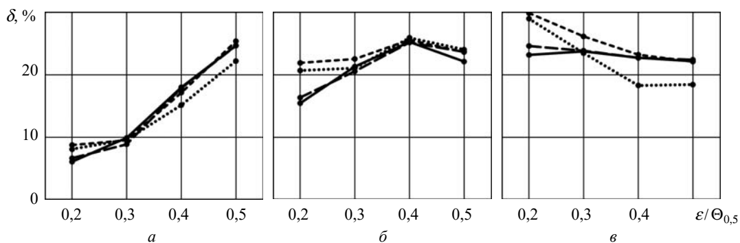
Рис. 7. Повышение точности измерения угла места при учете помех исключительно многолучевого распространения: a - \Delta f = 2 \% ; b - \Delta f = 4 \% ; v - \Delta f = 8 \% ; — — — — \rho_d = 0,36 ; - - - - \rho_d = 0,30 ; - · - · - \rho_d = 0,20 ; ······ \rho_d = 0,10
