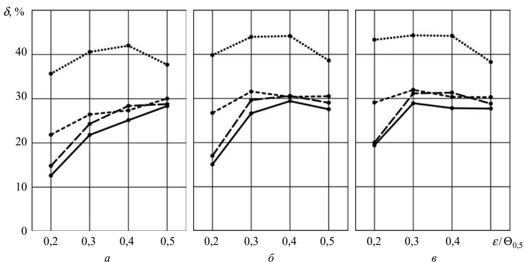
Рис. 8. Повышение точности измерения угла места при учете помех многолучевого распространения и тепловых шумов пеленгатора (ОСШ = 20 дБ): a - \Delta f = 2 \% ; b - \Delta f = 4 \% ; v - \Delta f = 8 \% ; — — — — \rho_d = 0,36 ; - - - - \rho_d = 0,30 ; - · - · - \rho_d = 0,20 ; ······ \rho_d = 0,10
