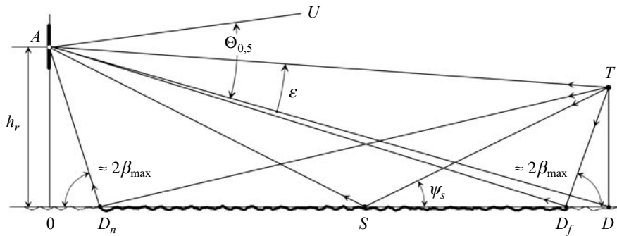
Рис. 1. Геометрия трассы
