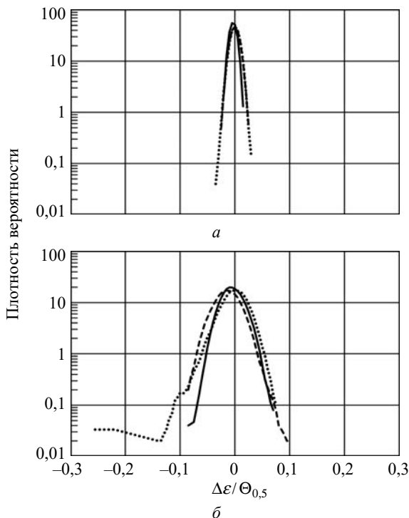
Рис. 2. Распределение ошибок измерения угла места при одночастотных измерениях, ОСШ = ∞: a – сильное зеркальное отражение; б – сильное диффузное отражение; - - - - - максимум поля; — — — — — промежуточная ситуация; ······ — минимум поля
