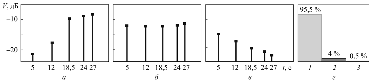
Рис. 6. Висотні залежності множника ослаблення для сигналів від п'яти відповідачів, розташованих на різних висоті: а – «зростаюча» залежність; б – «нейтральна» залежність; в – «спадна» залежність; г – гістограма
