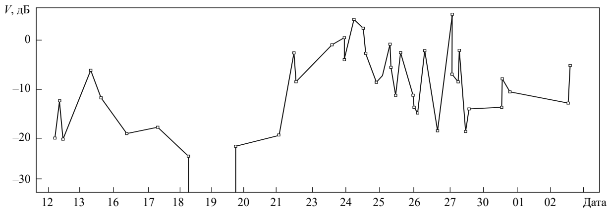
Рис. 5. Зміна середніх значень множника ослаблення на трасі 60 км (висота установки відповідача 27 м) у літній період (з 12 червня до 2 липня)
